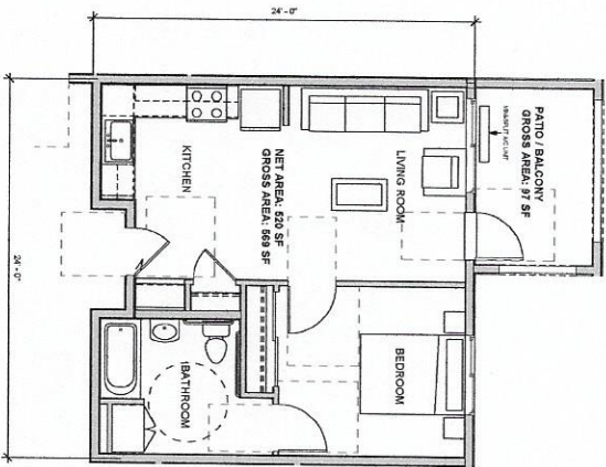
② TYPE B - 1BD 1BA SCALE: 1/4" = 1'-0"
